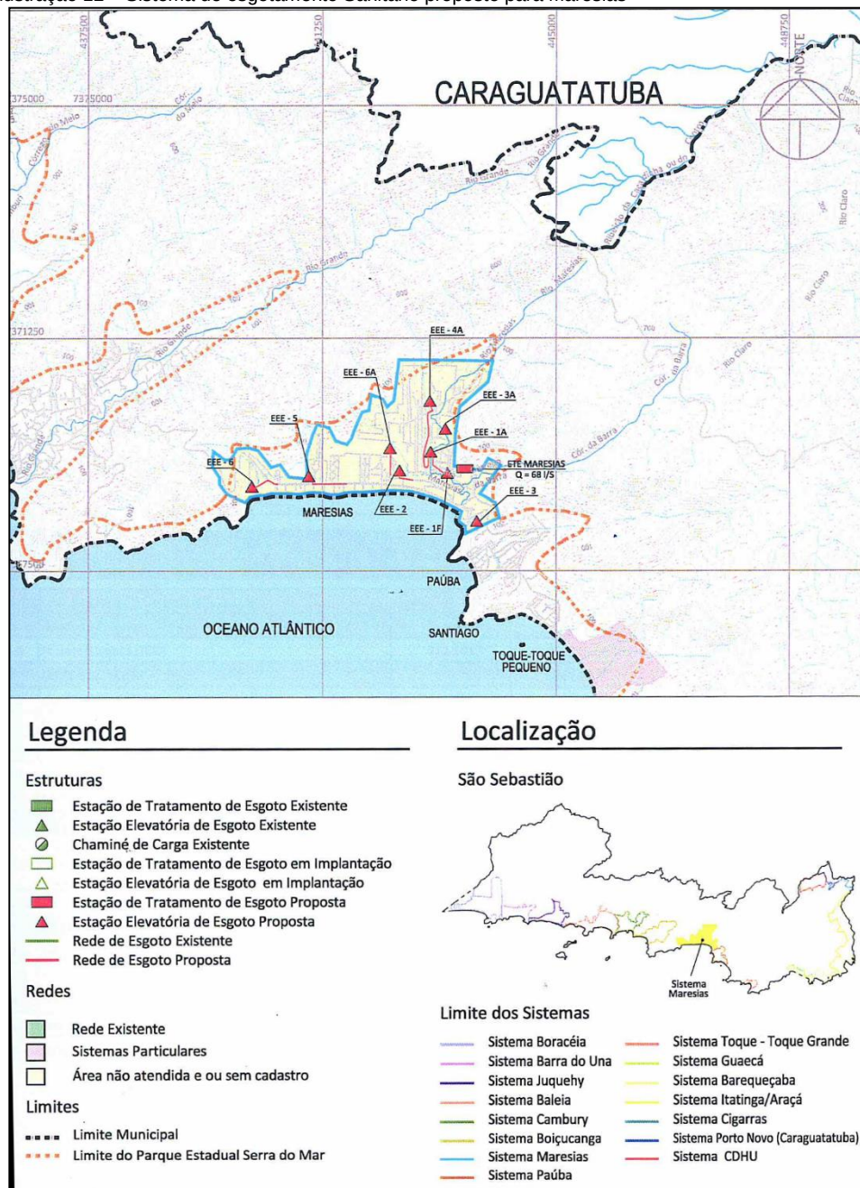
Ilustração 12 – Sistema de esgotamento Sanitário proposto para Maresias
