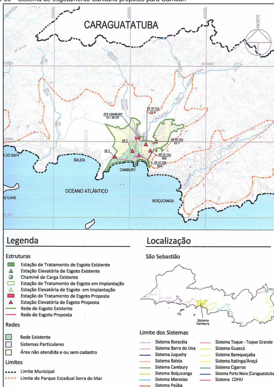
Ilustração 13 – Sistema de esgotamento Sanitário proposto para Camburi
